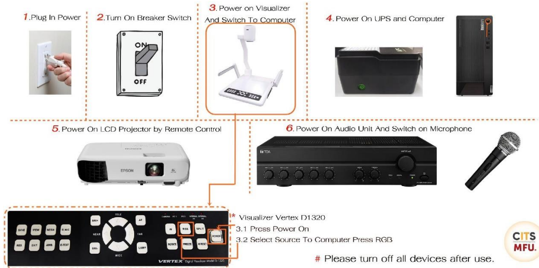
รูปแสดงการต่อพ่วงอุปกรณ์ภายในห้องเรียน แบบที่ 2
