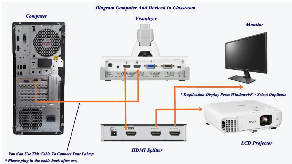
รูปแสดงการต่อพ่วงอุปกรณ์ภายในห้องเรียน แบบที่ 1
